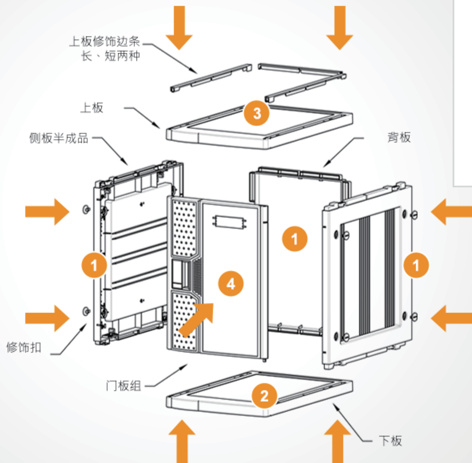
置物柜/分解图
